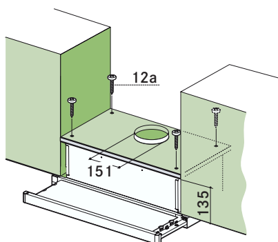
Montáž přes nosnou plochu
