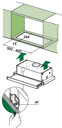
Montáž přes boční úchyty
