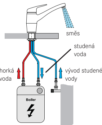
schéma zapojení beztlakové baterie – bez sprchy
