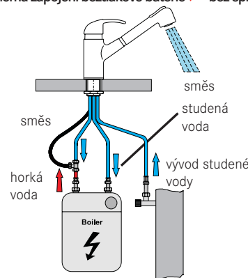
schéma zapojení beztlakové baterie – se sprchou
